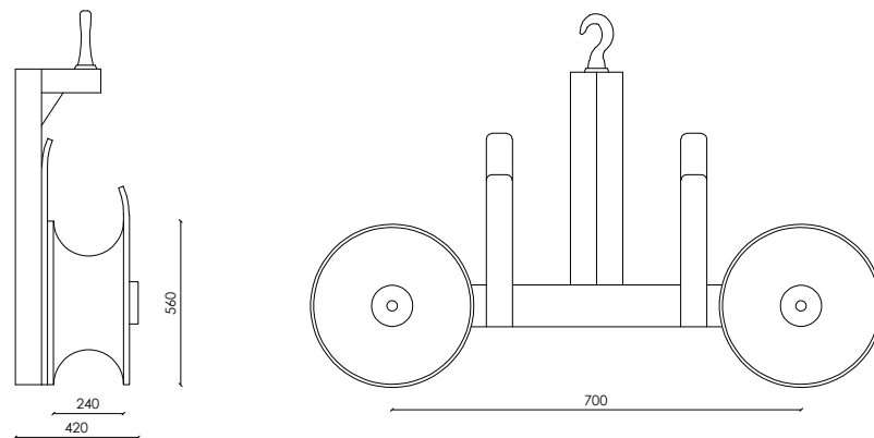
ROLDANA DOBLE Ø280mm
